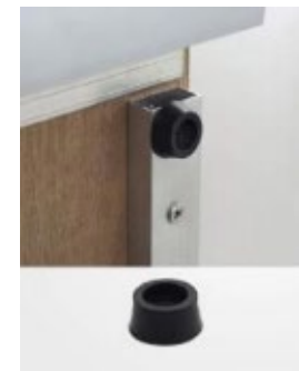
T-7 rubber stoppers 50 per bag, 1 per joist
